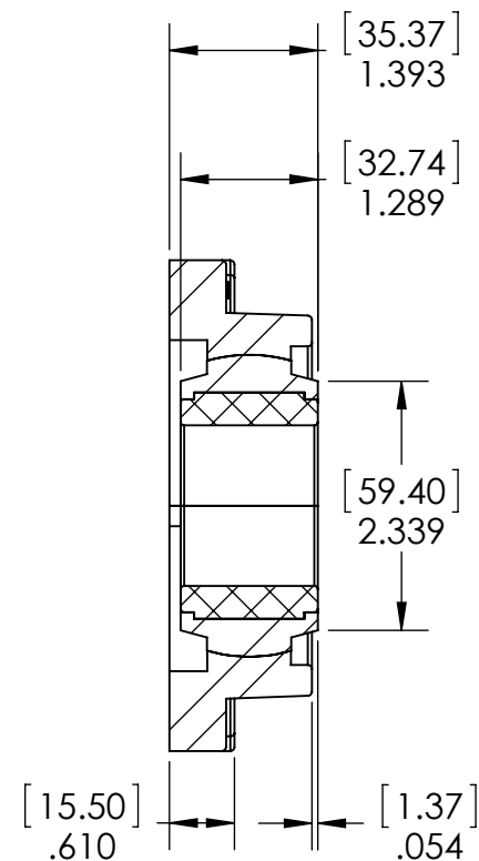
SECTION T-T SCALE 1 : 2
